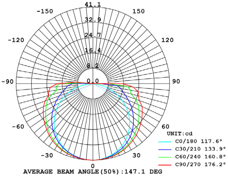
BLEU
