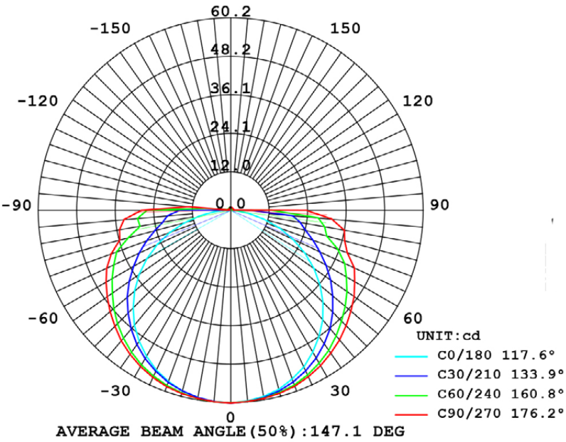
ROUGE
